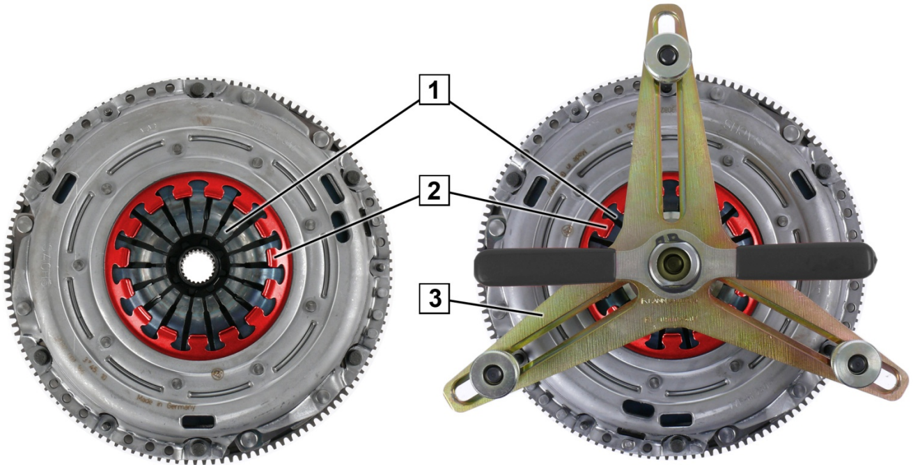
Sl. 1: Dodatna opruga
